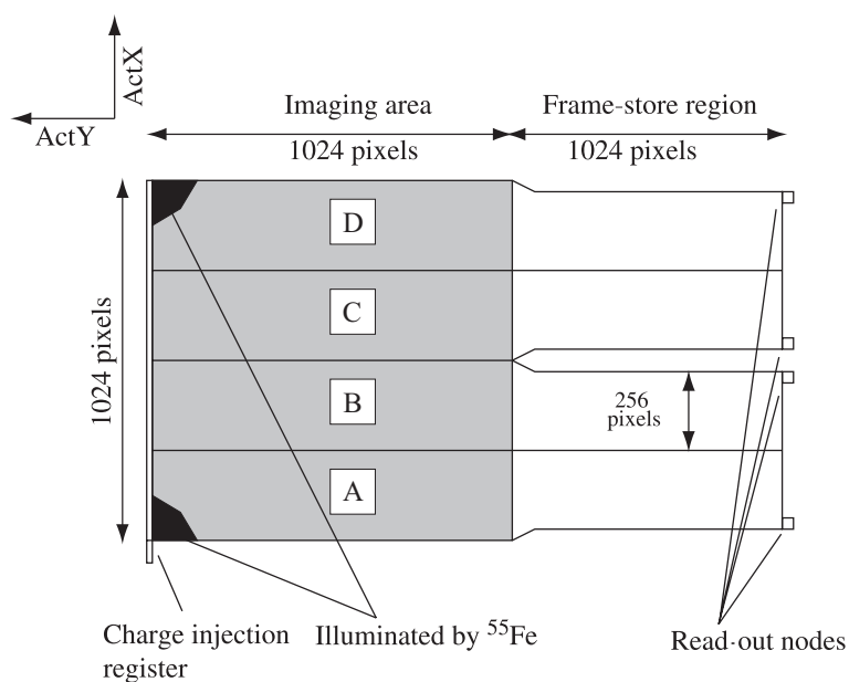
Fig. 5.11. —: Schematic view of the XIS CCD (Koyama et al. 2007a).
