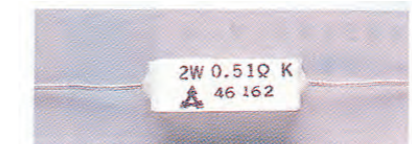
〈写真10〉セメント抵抗(電力用)：おもに巻き線抵抗体を難燃性ケースに収めたもの。安全性/実装性とも良好。
