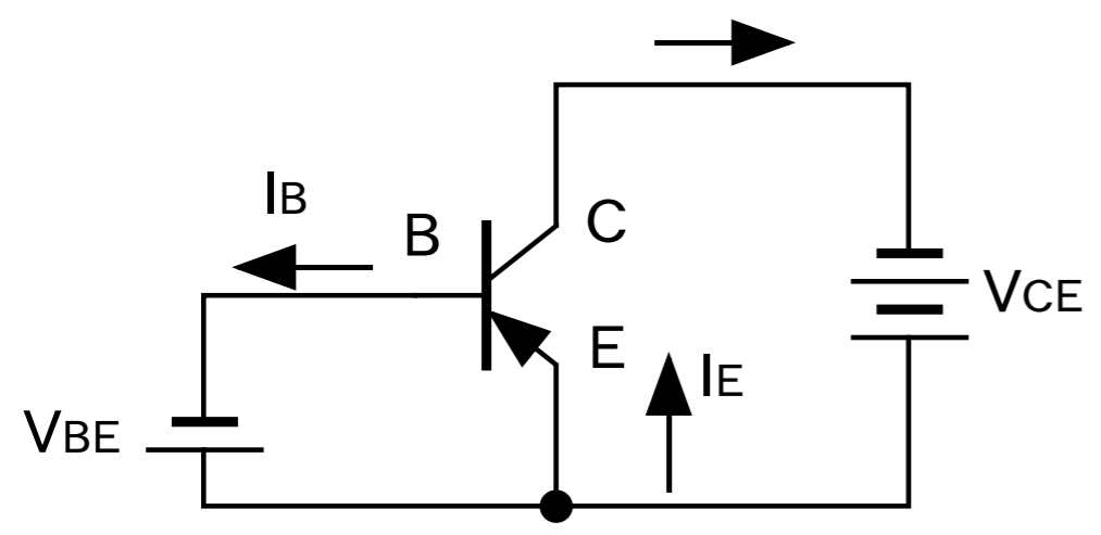
PNP型バイポーラトランジスタ
