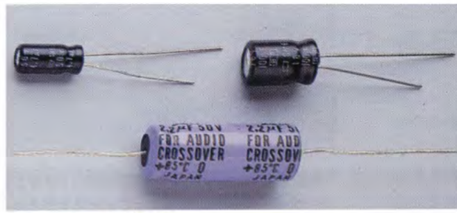
〈写真 16〉 無極性電解コンデンサ：誘電体は酸化アルミニウム。実用容量範囲は0.1 \mu ~100 \mu F。両極に酸化膜を付けたもの。
