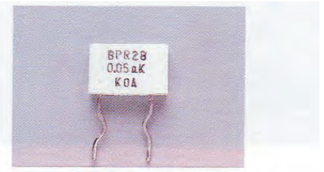
〈写真7〉金属板抵抗(低抵抗)：1 Ω 以下を得意とする抵抗。リード線抵抗の扱いに工夫が必要。
