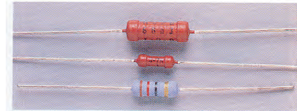
〈写真9〉酸化金属皮膜抵抗(電力用)：10 W 以内では特性もよく一般的。ディレーティングを考慮すること。
