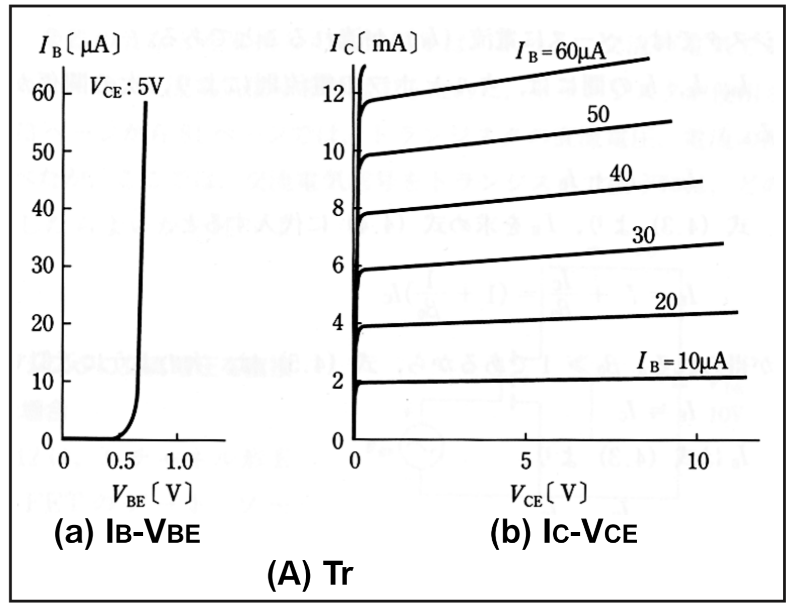
図 1.23: バイポーラトランジスタの特性.
