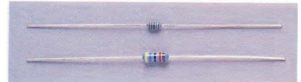
〈写真2〉厚膜金属皮膜抵抗(高精度)：安価で入手容易な焼結型の高精度抵抗。温度係数は±200 ppm程度。
