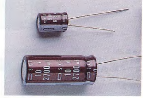
〈写真 13〉 高リプル電解コンデンサ：誘電体は酸化アルミニウム。実用容量範囲は10 \mu ~4700 \mu F。高域インピーダンス低減品。おもにスイッチング電源用。
