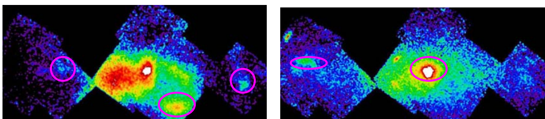
図 1：銀河中心付近 500×100 光年の高電離硫黄 (左) と鉄 (右) の特性 X 線分布。所々にある赤、黄色の塊 (ピンクの丸) が新たに発見された超新星残骸
